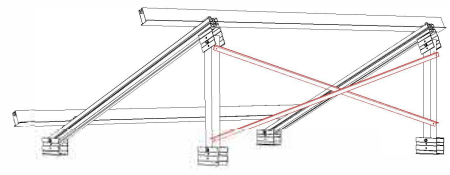
Arriostramiento para 2 triángulos
