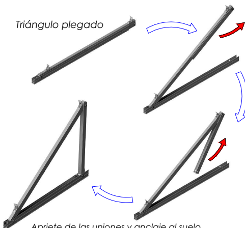
Apriete de las uniones y anclaje al suelo mediante tornillo de hasta M10
